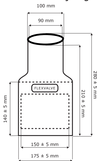
Slangetilslutning med 45° bøjning
