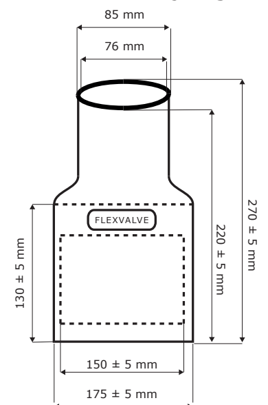
Slangetilslutning med 45° bøjning
