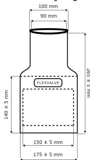
Slangetilslutning uden bøjning
