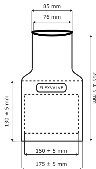
Slangetilslutning uden bøjning
